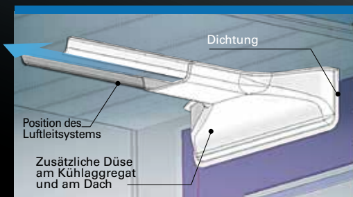
Patentiertes IAFO-System
